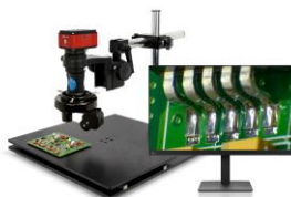
二维/三维高清视频显微镜 EC-S4
